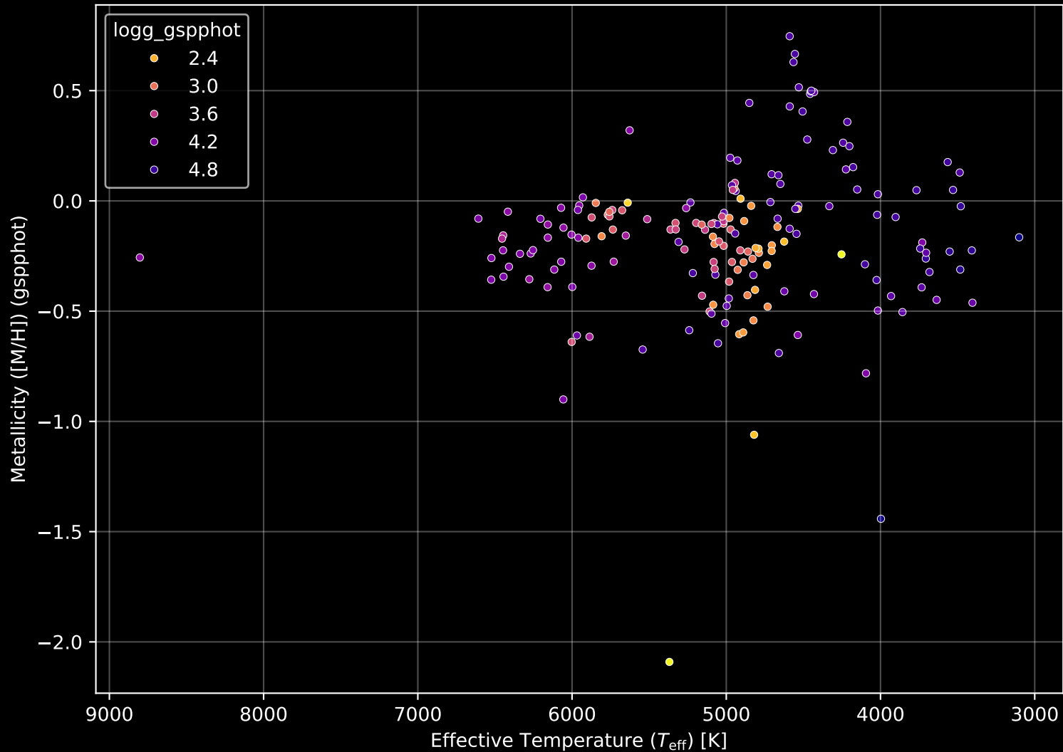
APOGEE DR17 Field: [110+60] Stellar Population Parameters (n= 182)
